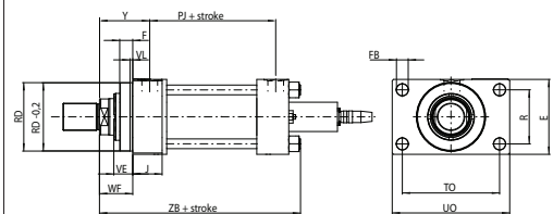
N (ISO ME5) = front flange
