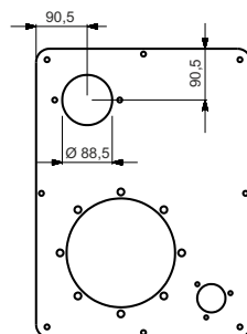
Кришка типу D / Кришка з вирізом під заливну горловину-сапун (FB), колокос (BH) та зливний фільтр (RF)
