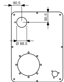
Кришка типу D / Кришка з вирізом під заливну горловину-сапун (FB), колоккол (ВН) та зливний фільтр (RF)
