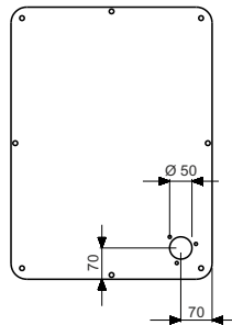
Кришка типу В / Кришка з вирізом під заливну горловину-сапун (FB)
