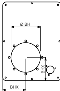
Кришка типу С / Кришка з вирізом під заливну горловину-сапун (FB) та колокос насоса/електродвигуна (BH)
