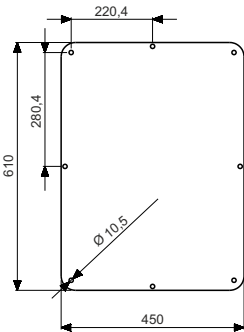
Кришка типу А / Глуха кришка
