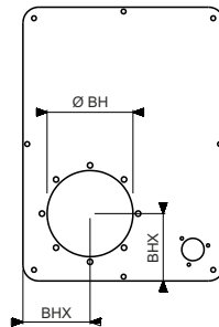
Кришка типу С / Кришка з вирізом під заливну горловину-сапун (FB) та колоккол насоса/електродвигуна (ВН)
