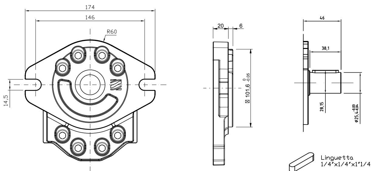
GR55 - TYPE / TIPO SAEB-AC
