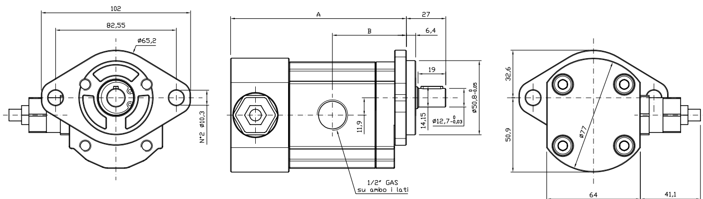
GR28 - TYPE / TIPO SAEA-A - AC (with safety valve/con valvola di massima)
