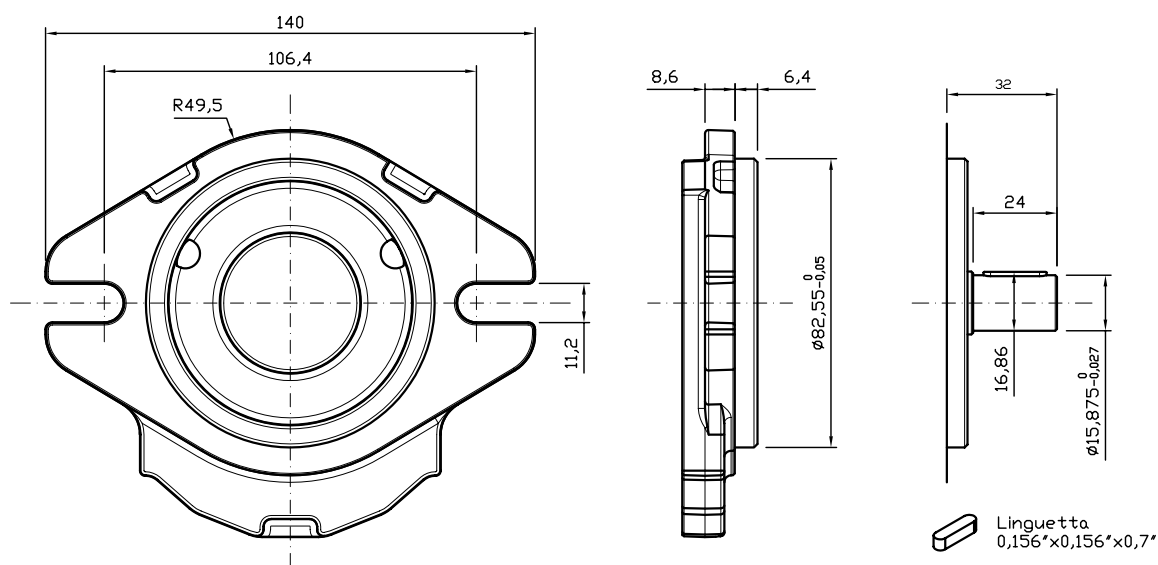
GR33 - TYPE / TIPO SAEA-AC
