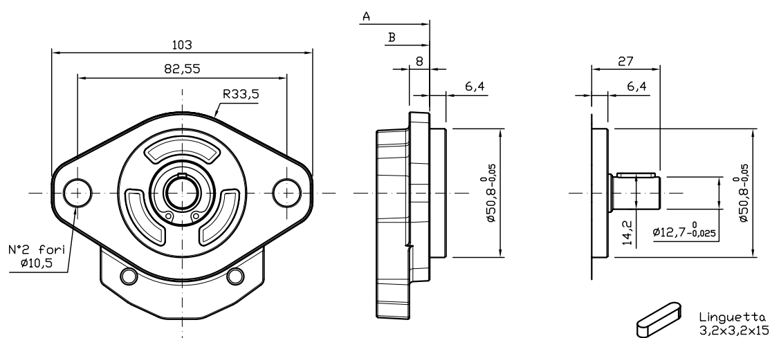
GR28 - TYPE / TIPO SAEA-A - AC
