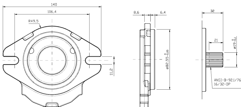
GR38 - TYPE / TIPO SAE-T11
