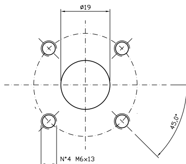
Type Q / Tipo Q
