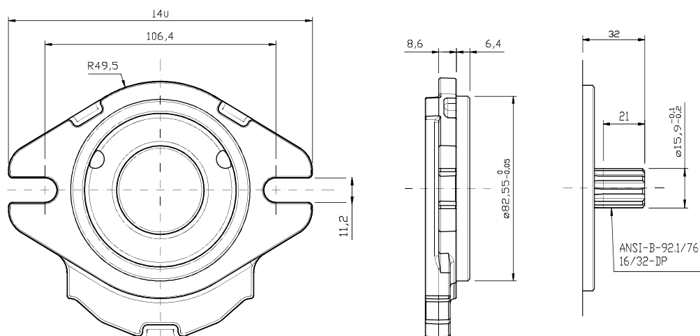
GR38 - TYPE / TIPO SAEA-T9
