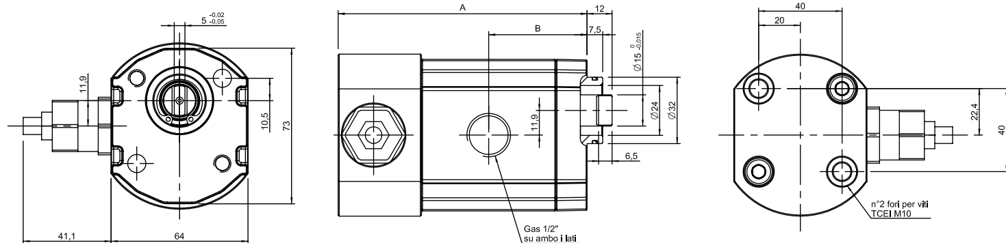
GR28 - TYPE / TIPO 1K-GL54 (with safety valve / con valvola di massima)
