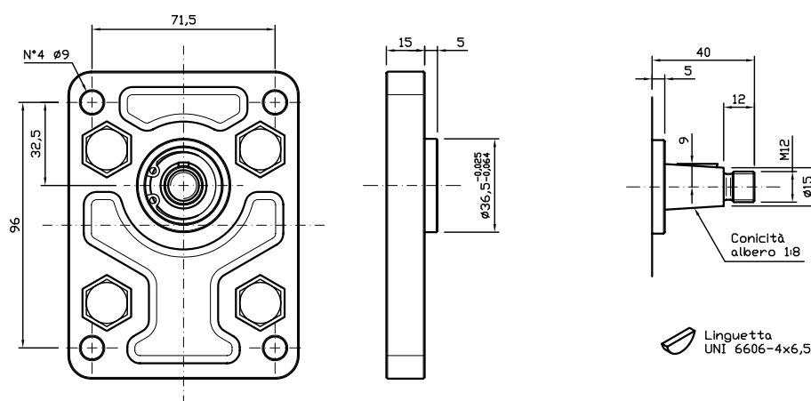
GR38 - TYPE / TIPO 2-C4
