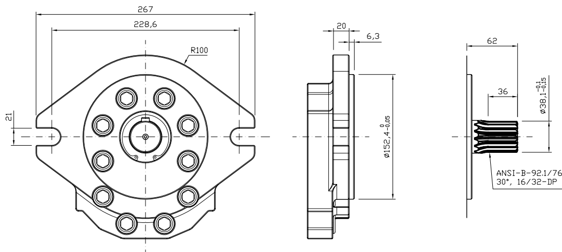
GR72 - TYPE / TIPO SAED-T23
