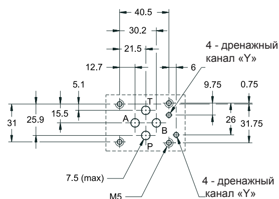
МОНТАЖНАЯ ПОВЕРХНОСТЬ ФРМ3
