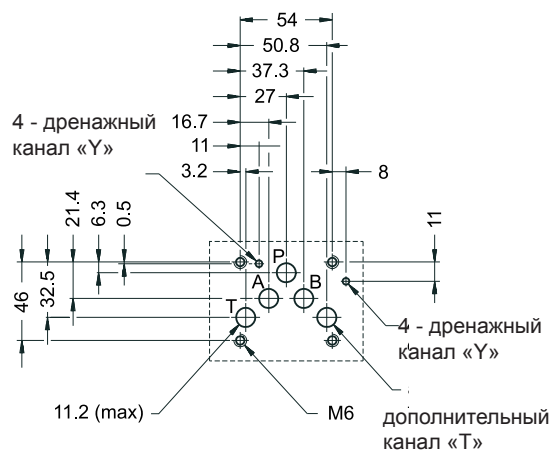
МОНТАЖНАЯ ПОВЕРХНОСТЬ ФРМ5
