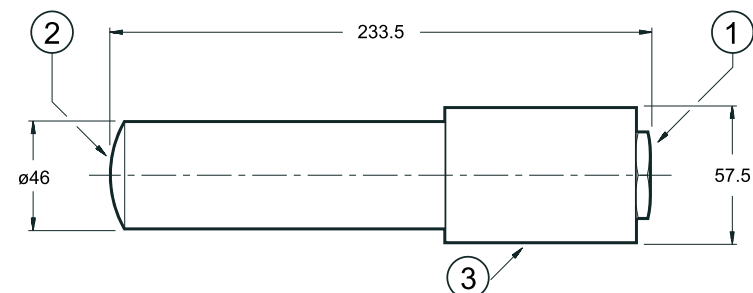
МОНТАЖНАЯ ПОВЕРХНОСТЬ ФРМ3
