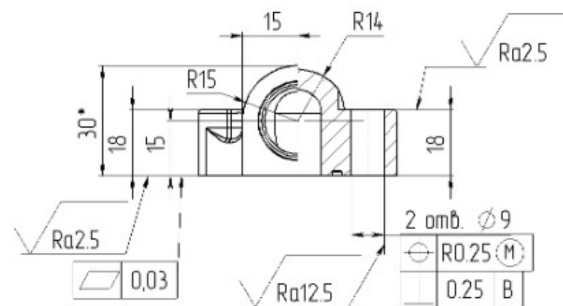
СІЧЕННЯ Б-Б
