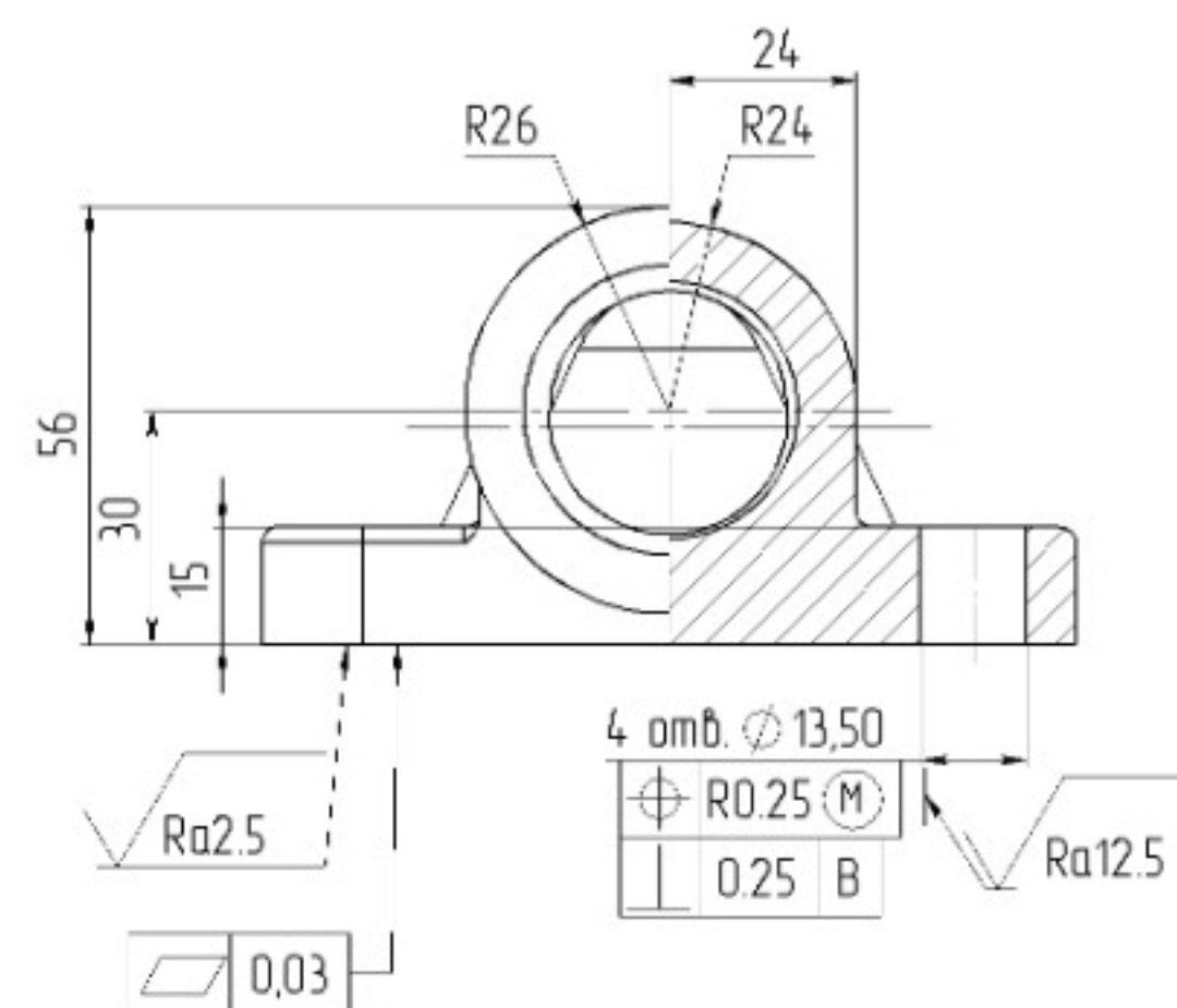
СІЧЕННЯ Б-Б
