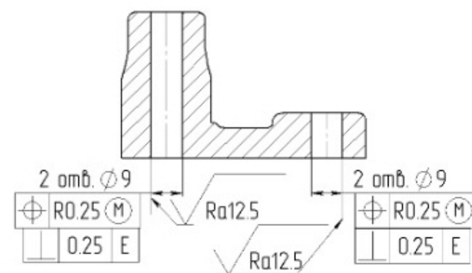
СІЧЕННЯ В-В
