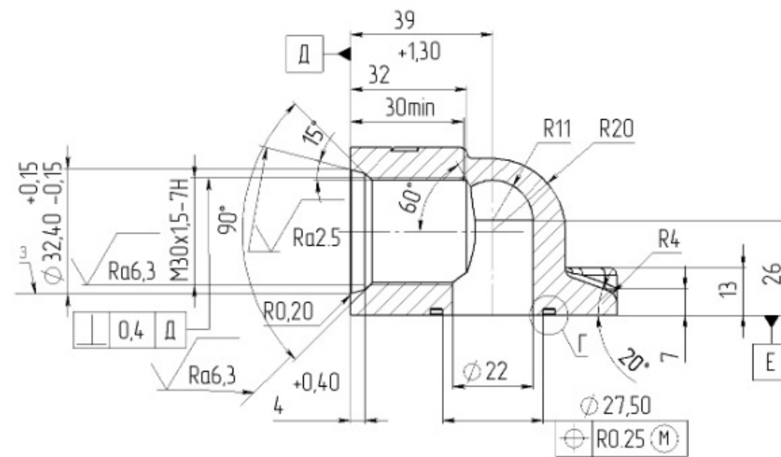
СІЧЕННЯ А-А
