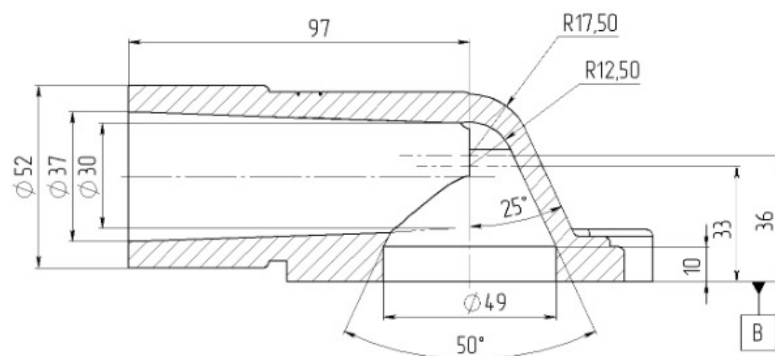
СІЧЕННЯ А-А
