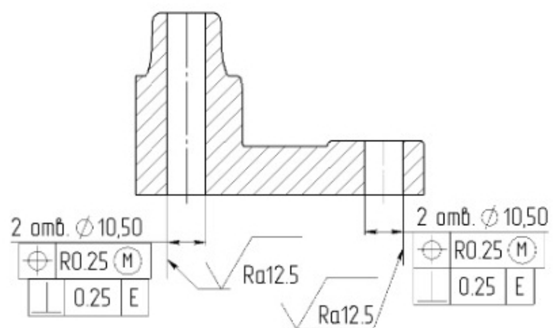
СІЧЕННЯ В-В
