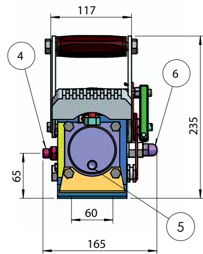
Einbaulage - Mounting Position:
