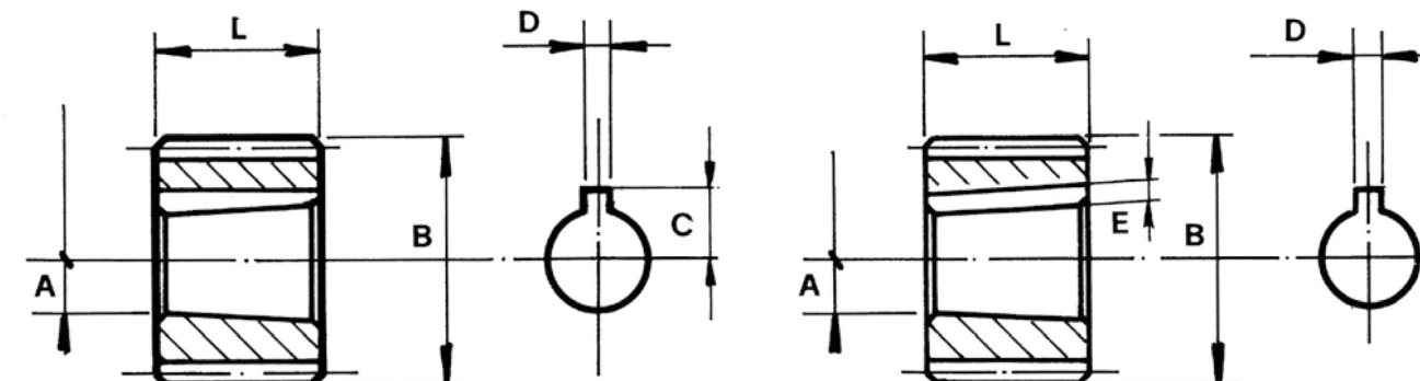
Conicità 1:5 - Conicité 1:5 - Taper ratio 1:5 - Keilneigung 1:5
