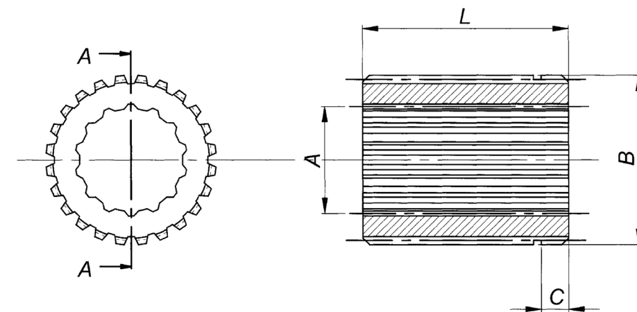
SEZ.: A-A
