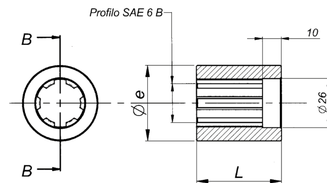
SEZ.: B-B
