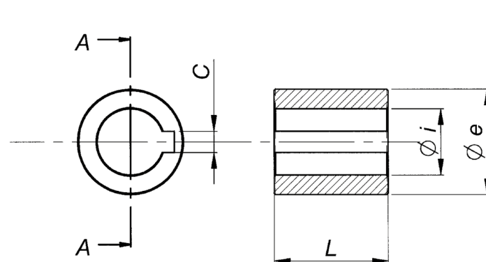
SEZ.: A-A
