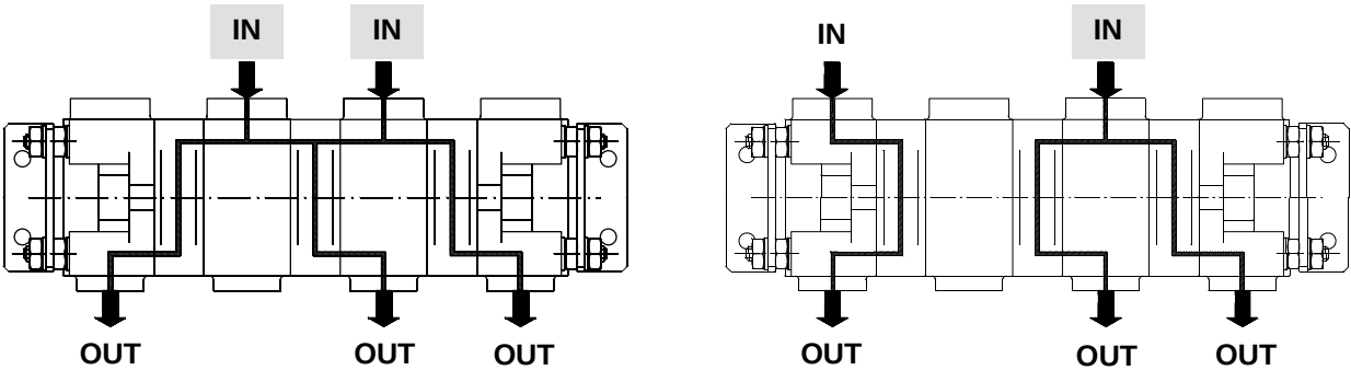
Equalizzatore di flusso con sezione motore. Flow equalizer with motor section.
