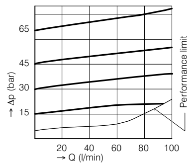
\Delta p -Q characteristic DVPA-RV-1-10-...L
